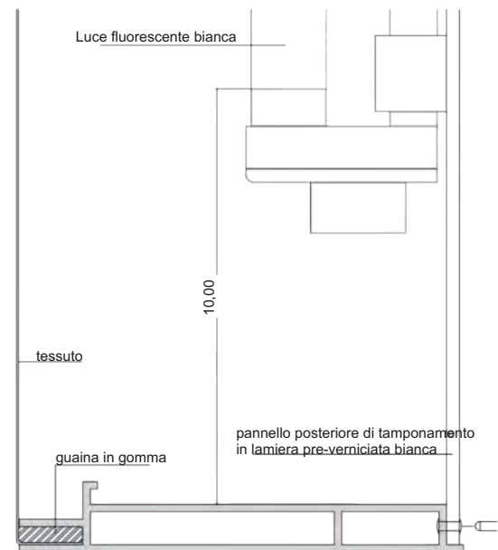
Schema per illuminazione con tubi fluorescenti
