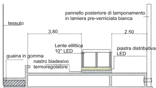
Schema per illuminazione a LED
